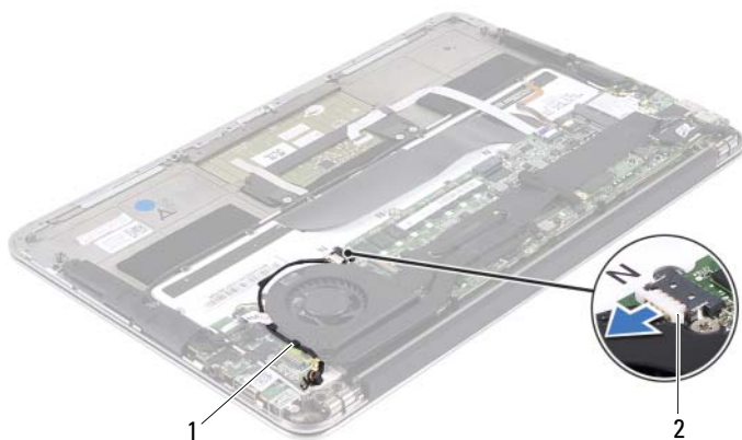
1 布线导向器
